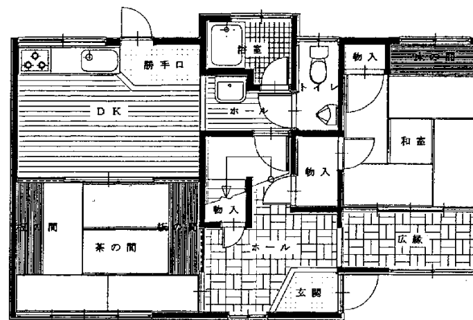
1階平面図
