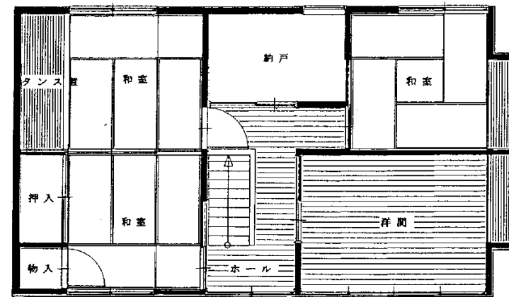
2階平面図
